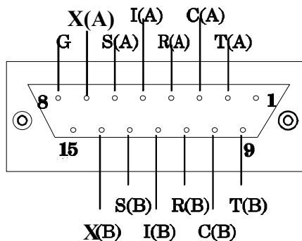
Connecteur ISO 4903 - Vue côté contacts.
